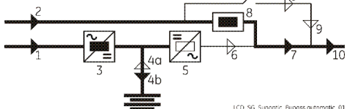
Мнемосхема на первом ИБП
