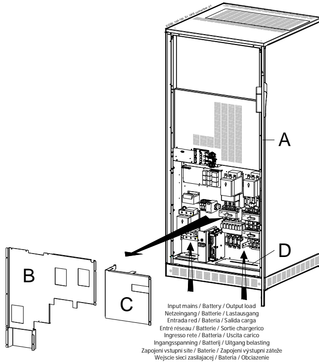
Рис. 5.6-2 SG-CE Series 100 – 120 кВА PurePulse® Доступ к силовым шинам
