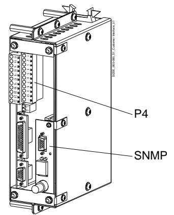
Рис. 2.1-5 Блок интерфейсов
