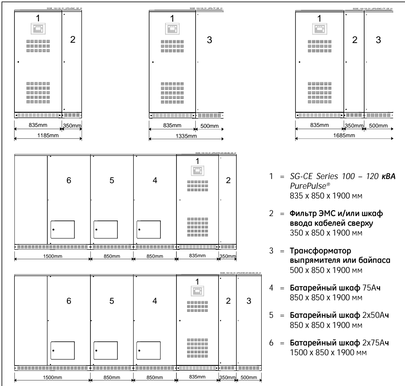
Вес ИБП SG-CE Series 100 – 120 кВА PurePulse® и опций
