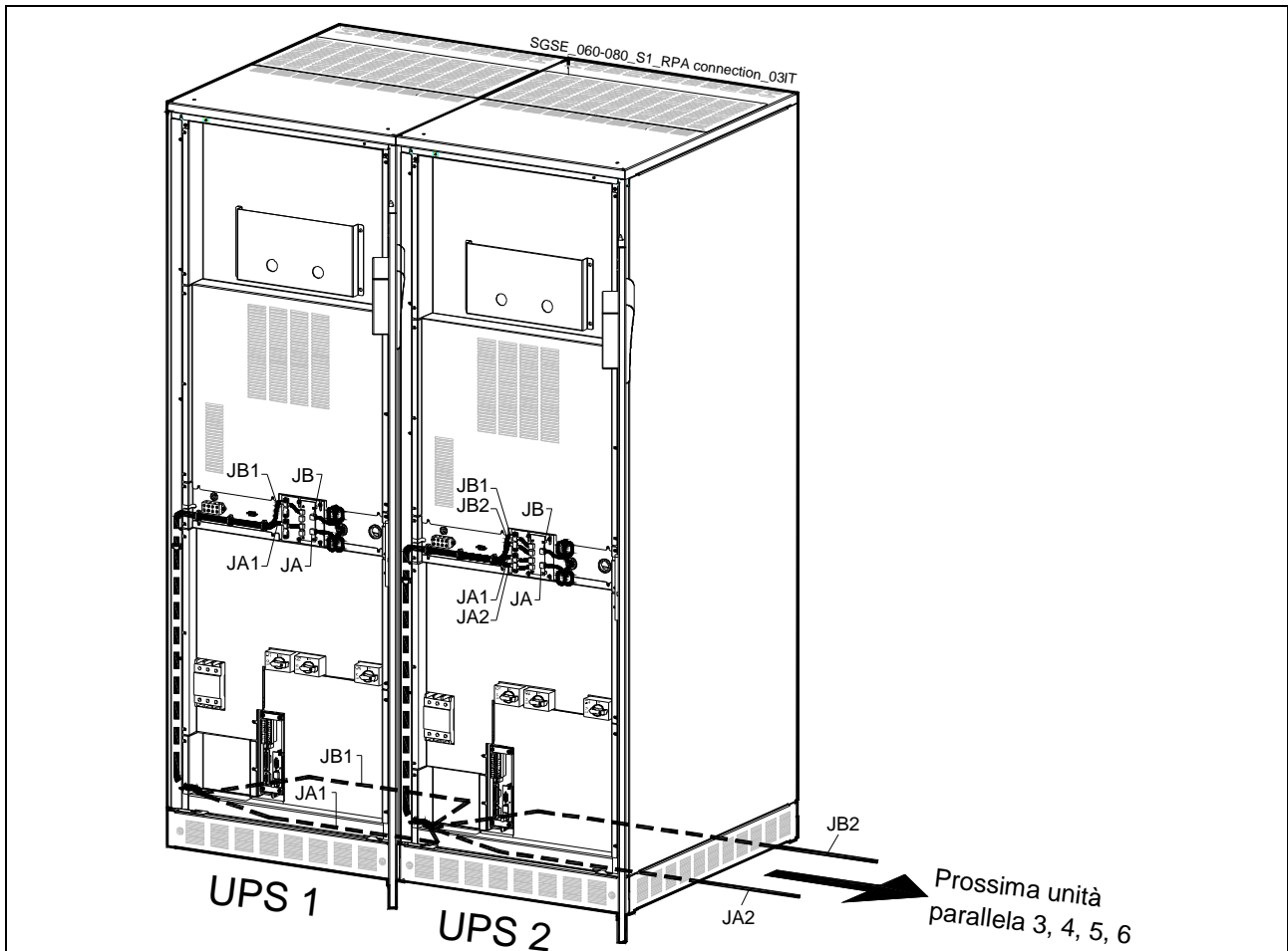
Рис. 5.9.3-3 Прокладка кабелей шины управления
