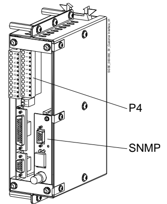
Рис. 2.2-5 Блок интерфейсов
