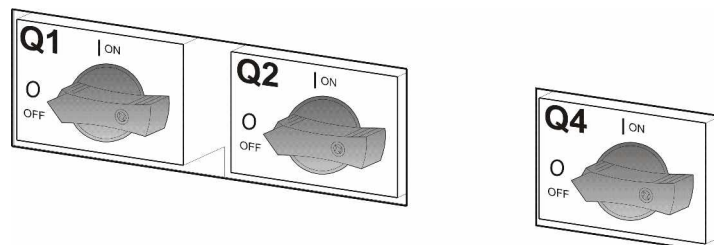
Рис. 2.2-6 Ручные переключатели
