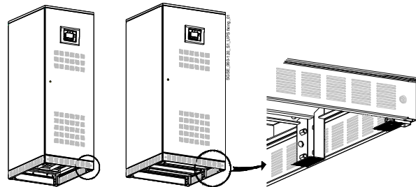
Рис. 5.4.1-4 Крепление шкафа ИБП к полу
